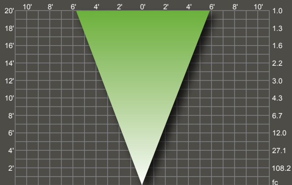
20W PAR36: HP36/WFL20/HX
