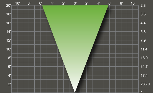
35W PAR36: HP36/WFL35/HX
